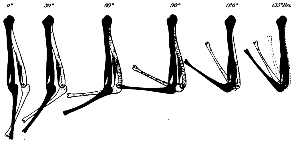
Anfang der Beugebewegung des unbelasteten Arms bei alleiniger Contraction eines eingelenkigen Beugemuskels des Ellbogengelenks für verschiedene Ausgangsstellungen.
